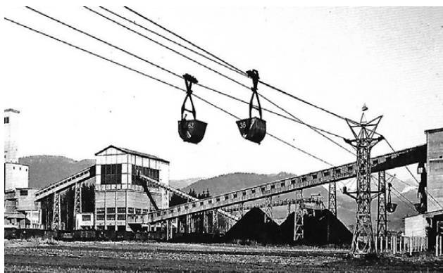
Viseča žičnica za prevoz premoga do deponije leta 1957
