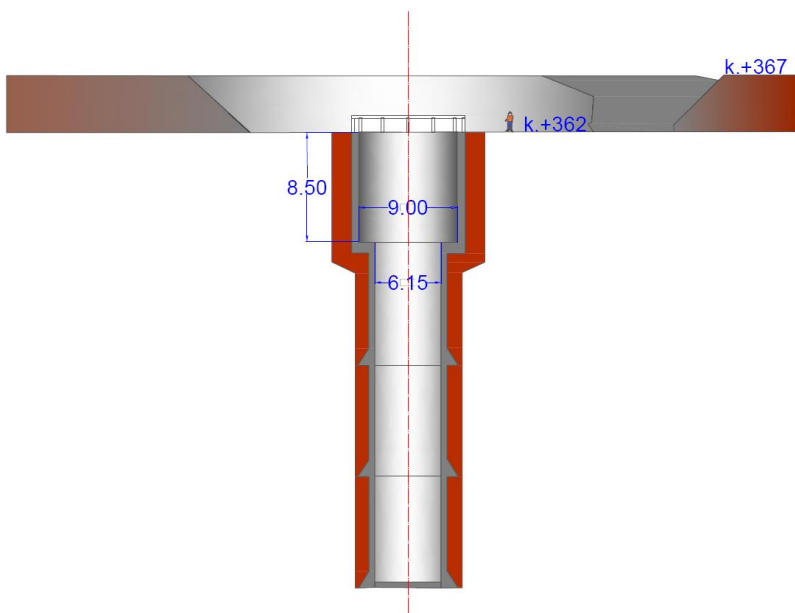
Slika 4: 3D-skica prečnega prereza Zračilnega jaška NOP II z okolico.
