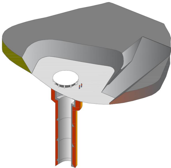
Slika 2: 3D skica Zračilnega jaška NOP II z okolico.
